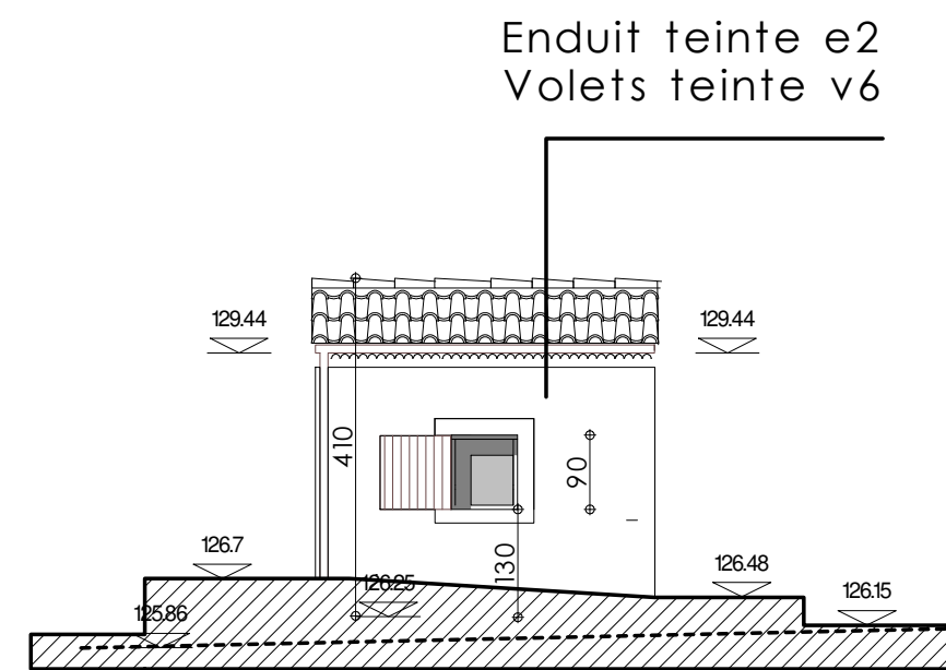
FACADE SUD EST
