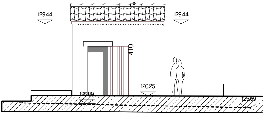
FACADE NORD OUEST
