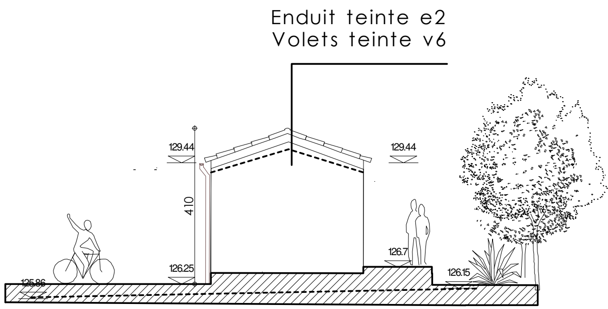
FACADE SUD OUEST
